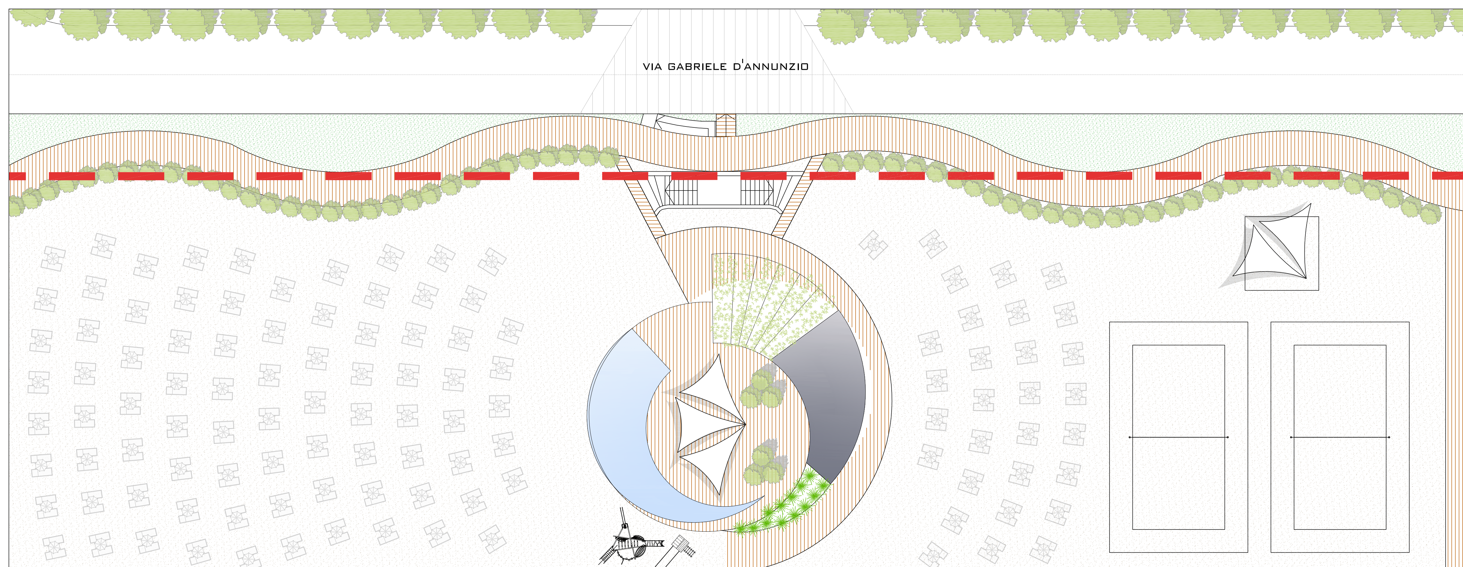
DETTAGLIO LUNGO MARE E SERVIZI SPIAGGIA PLANIMETRIA SCALA 1:200
