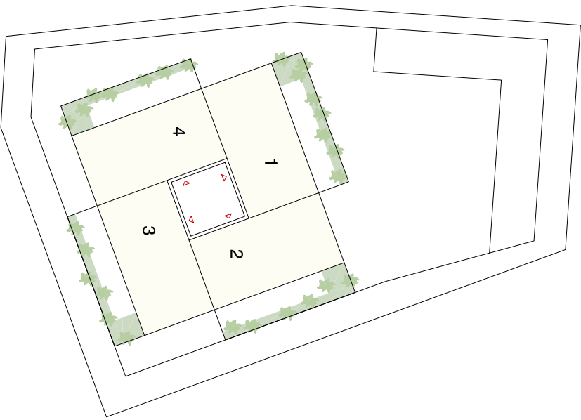
PIANTA PIANO TIPO RESIDENZE
